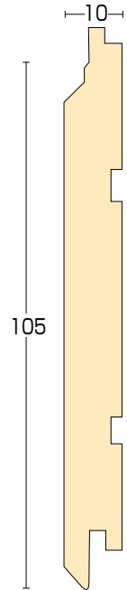
本実目透し加工 (エンドマッチ加工)
