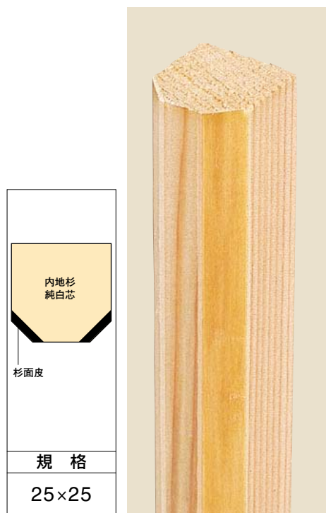
品名：12-4 白面皮天井竿
