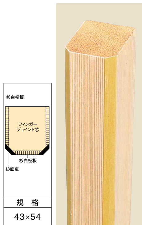
品名：12-6 白面皮棟木
