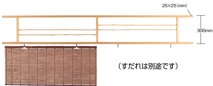
107-2 簾取付材(晒竹) ※黒竹も出来ます。
