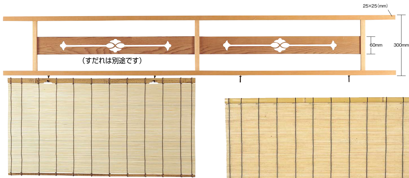
107-1 簾取付材(ランマ)
