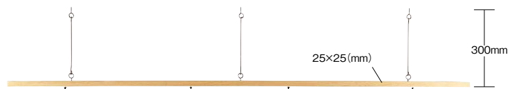
107-4 簾取付材(銅棒カギ式)
