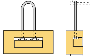
花蔓釘は足を割って埋木をして 掛け雨戸の上框に仕込む
