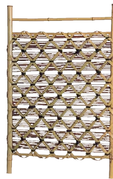
品番： 28-7 品名：晒竹萩入枝折戸 巾×高さ/尺(mm) 枚単価 2.0×3.5(600×1050) ¥29,500 2.3×3.5(690×1050) ¥31,000 2.5×3.5(750×1050) ¥32,000
