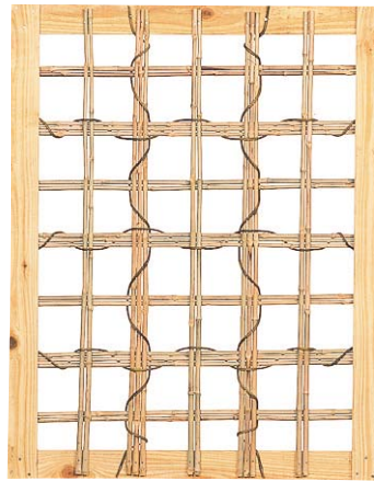
品番： 24-9 品名：木枠寒竹下地角窓
